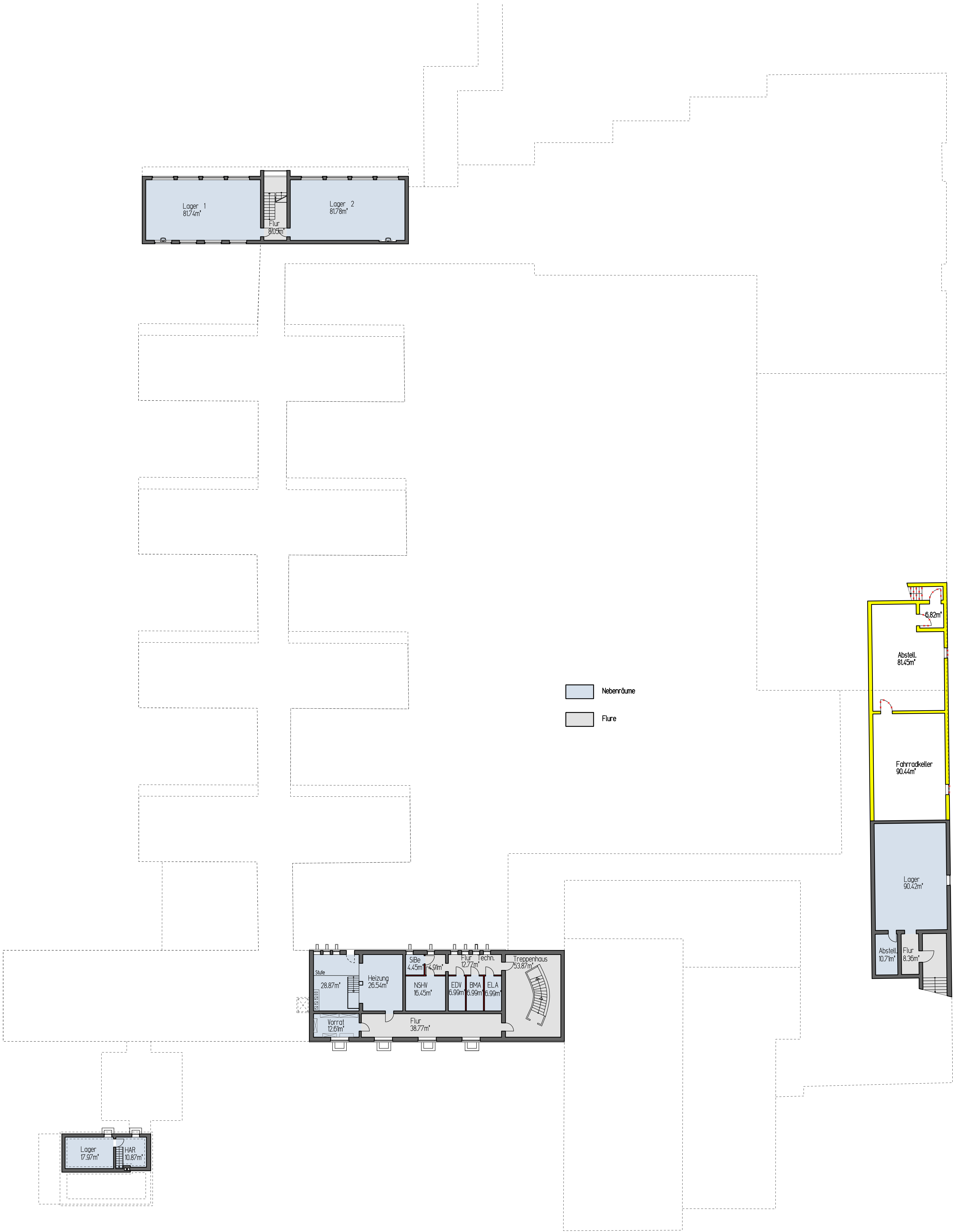
KELLERGEOSCHOSS M 1:200
