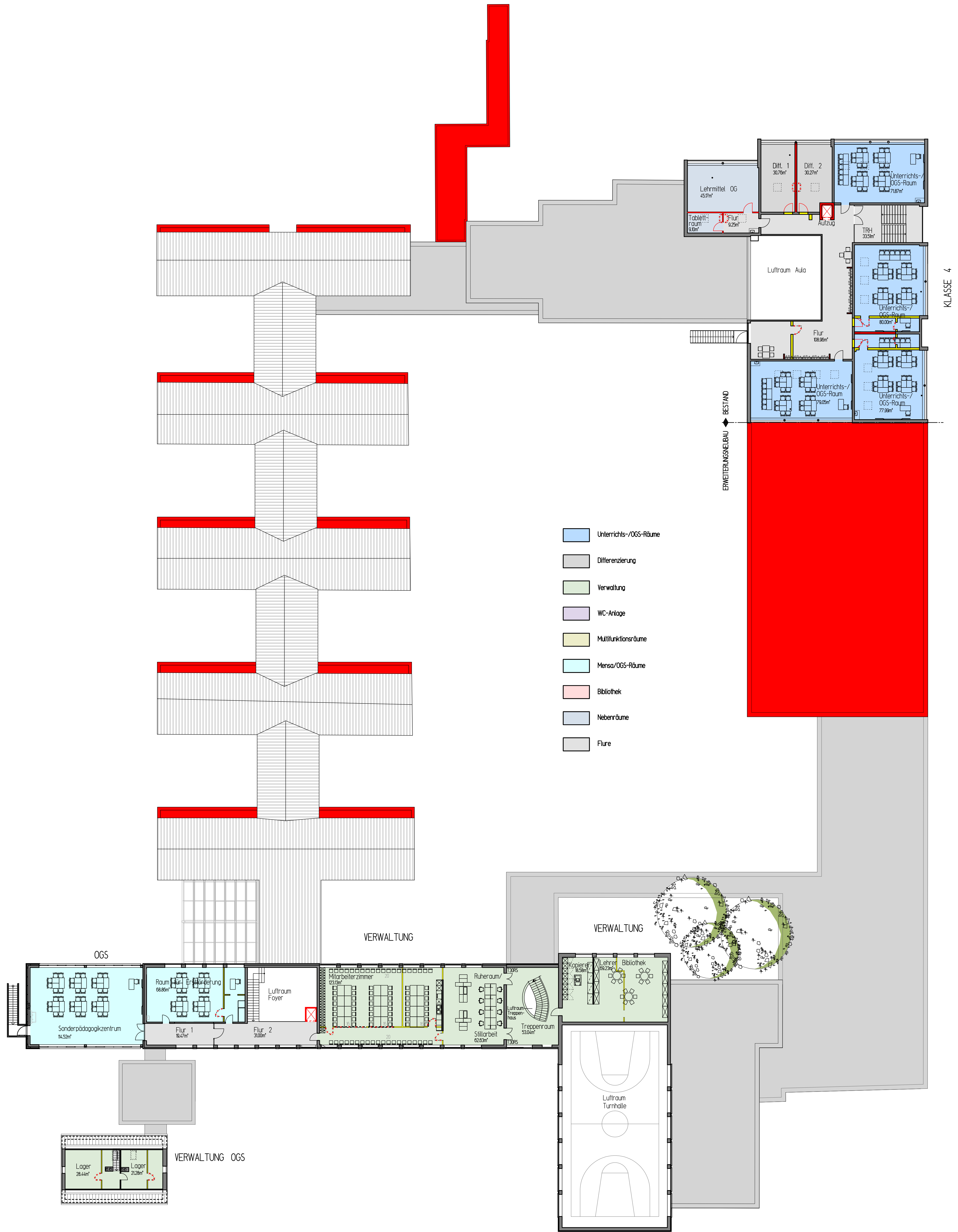
OBERGESCHOSS VARIANTE A UMB M 1:200 00 VI um
