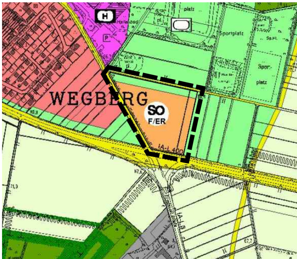
Abbildung 4 Darstellungen des Flächennutzungsplans im Plangebiet Stadt Wegberg
