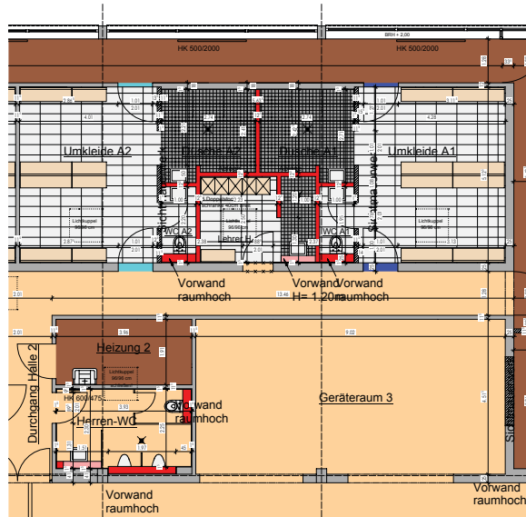
Detail Umkleiden und Duschräume M1.50
