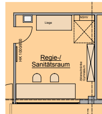
Detail Regie-/Sanitätsraum M1.50
