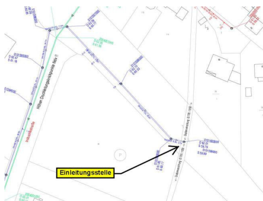
Einleitungsstelle
