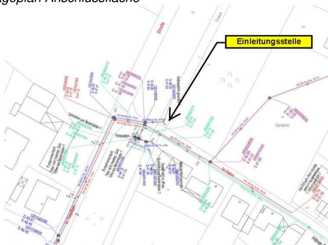
Einleitungsbauwerk
