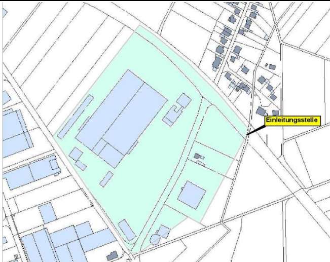
Lageplan Anschlussfläche
