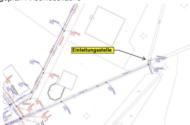
Einleitungsstelle
