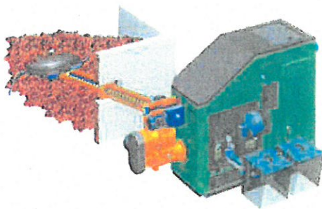
Bild: Hackschnitzelheizung
